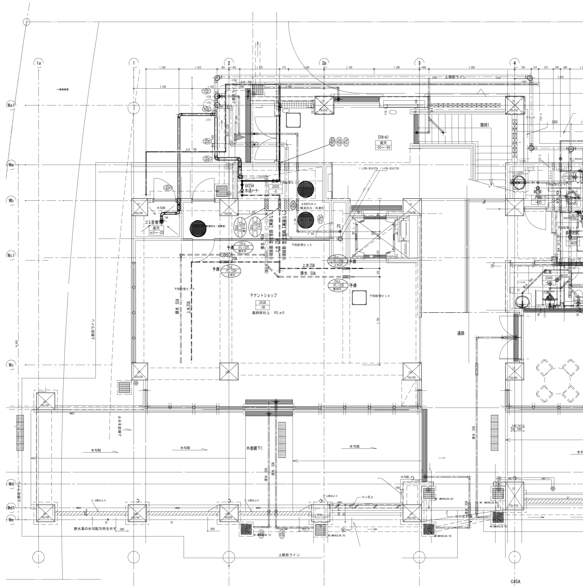
西棟 ショップ衛生配管平面図
