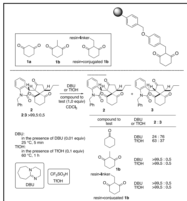
図 1. 環状 1,3-ジオン誘導体とその酸および塩基による異性化抑制への応用
