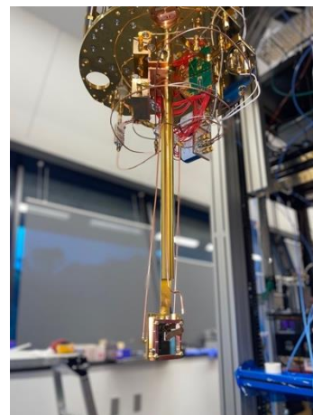
図 1. 希釈冷凍機に取り付けられたテストデバイス。このデバイスは約 10 ミリケルビン（約マイナス 273°C）まで冷却される。
