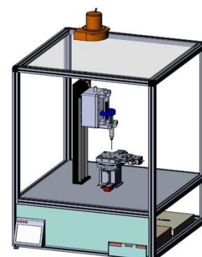
図 2. ハイブリッド加工技術の 3D-CAD 設計
