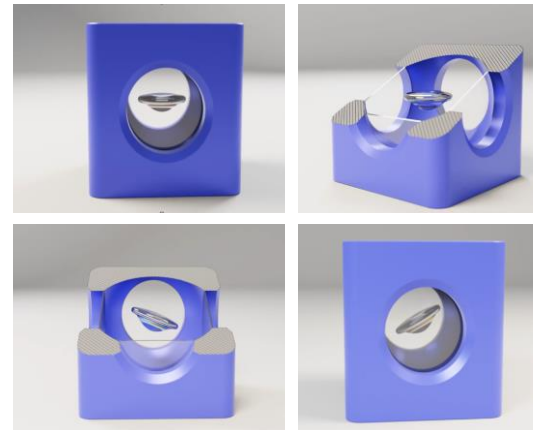
図 2：焦点距離、ピッチ、ヨーを変化させた、さまざまな構成の磁気可変レンズの概略図。形状は球面収差を補正している。
